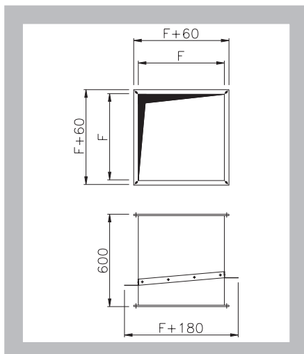
Рис. 13: Кровельный элемент
