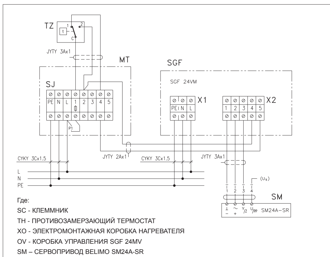
Рис. 20: Схема подключения противомерзающего термостата к водогрейному нагревателю с камерой смешивания (проведение .57), регулируемой коробкой SGF 24MV
