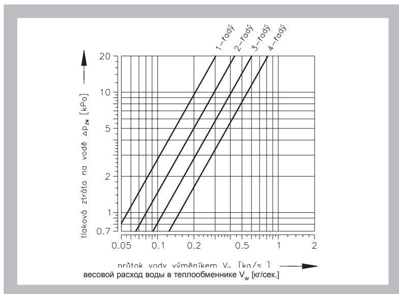
Рис. 5: Потери напора воды – модель 1
