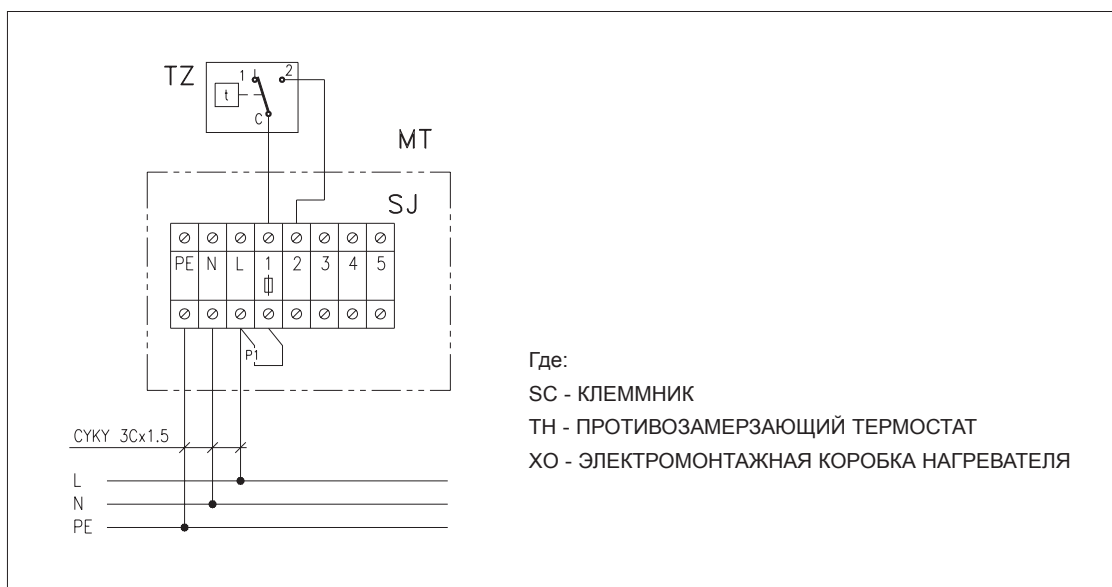
Рис. 19: Схема подключения противомерзающего термостата к водогрейному нагревателю
