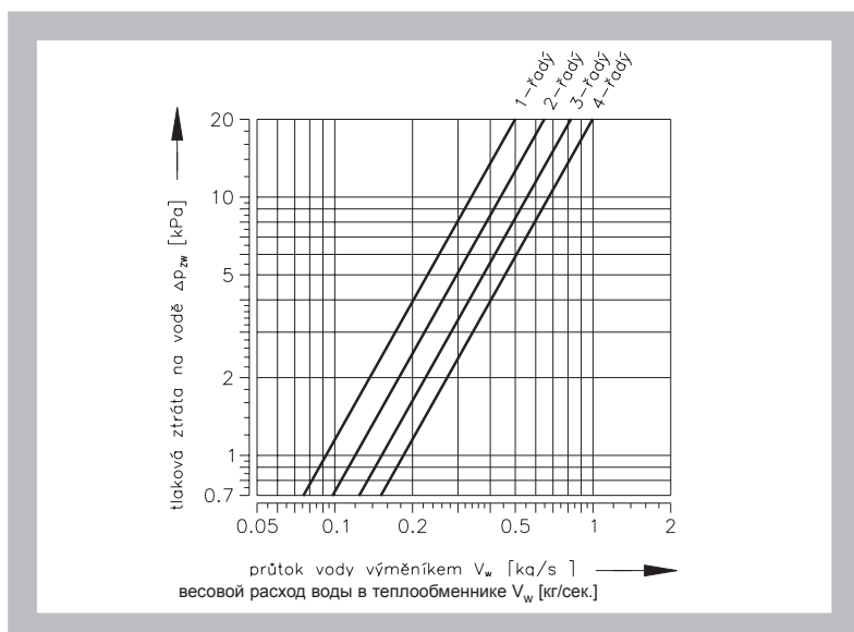
Рис. 6: Потери напора воды – модель 2
