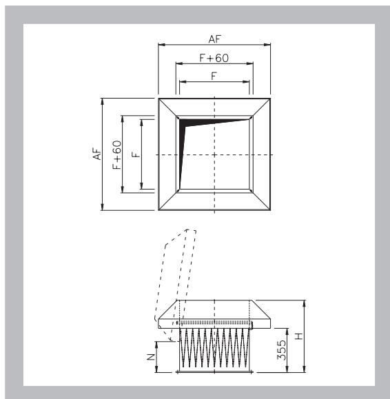
Рис. 14: Кровельный колпак
