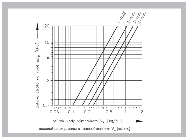
Рис. 7: Потери напора воды – модель 3
